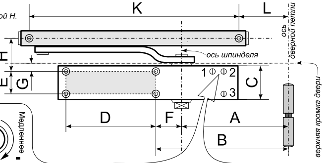
Рисунок 3. Монтаж с тягой H. (Правая дверь)
